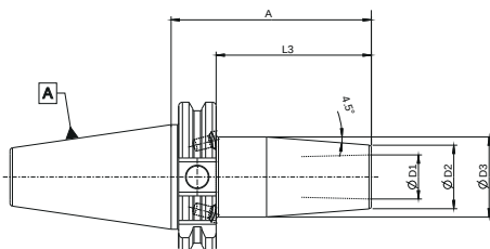
TMG14-85-AD40
